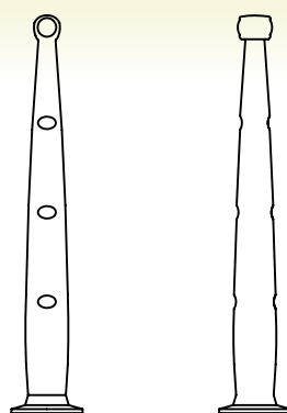
Arona h 1.000 mm - Ø 180 mm
