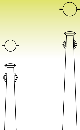
Philippi 670 h 670 mm · Ø 116 mm
