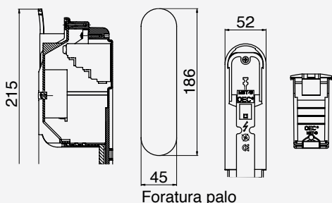
Foratura palo
